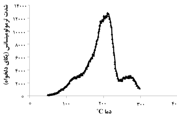
شکل ۴. شکل منحنی درخندگی قرص دزیمتر LiF:Mg,Ti
