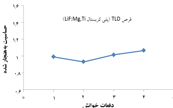
شکل ۳. بررسی ثبات پاسخ قرص دزیمتر LiF:Mg,Ti با دفعات خوانش.
