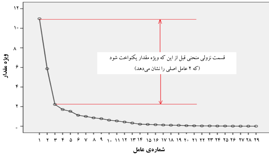
شکل ۴. نمودار اسکری.
