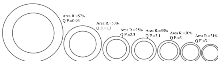
شکل ۱. کاهش سطح مقطع‌ها و ضریب‌های Q در مراحل مختلف نورد کاری ۶ مرحله‌ای.
