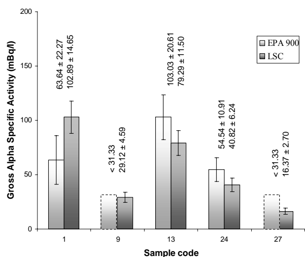
شکل ۲- نمودار مقایسه نتایج میزان پرتوزایی آلفا کل با دو روش LSC و EPA 900
