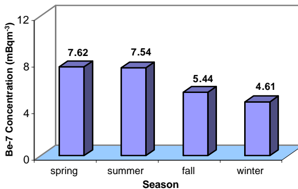
شکل ۳- تغییرات فصلی غلظت پرتوزایی ^7\text{Be} ، سال ۱۳۸۱، ایستگاه تهران.
