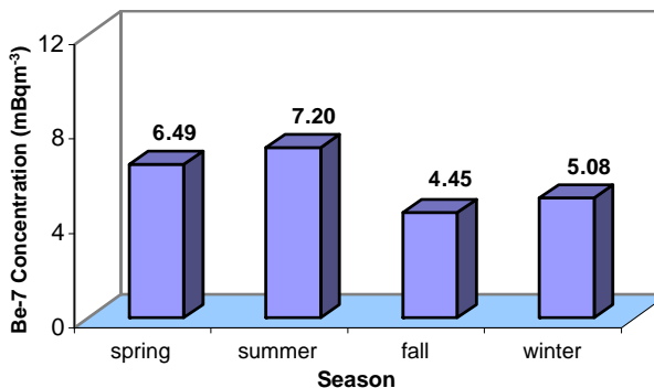
شکل ۴- تغییرات فصلی غلظت پرتوزایی ^7\text{Be} ، سال ۱۳۸۲، ایستگاه تهران.
