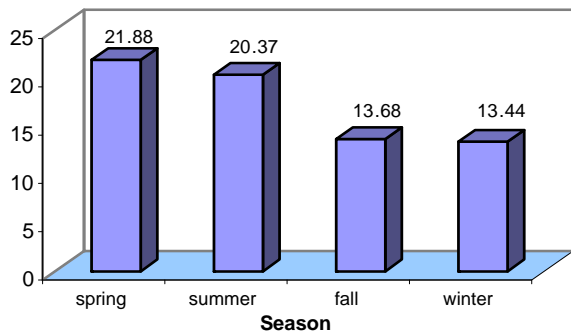
شکل ۷- متوسط تغییرات فصلی غلظت پرتوزایی ^7\text{Be} ، سالهای ۱۳۷۸ تا ۱۳۸۲، ایستگاه زاهدان.
