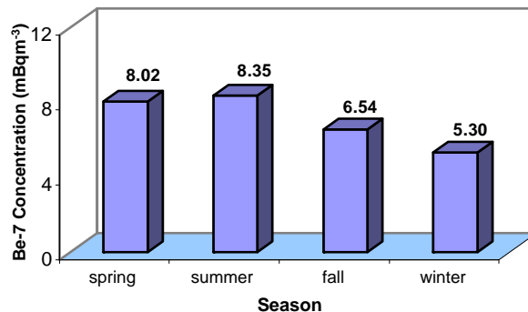
شکل ۵- تغییرات فصلی غلظت پرتوزایی ^7\text{Be} ، سال ۱۳۸۳، ایستگاه تهران.
