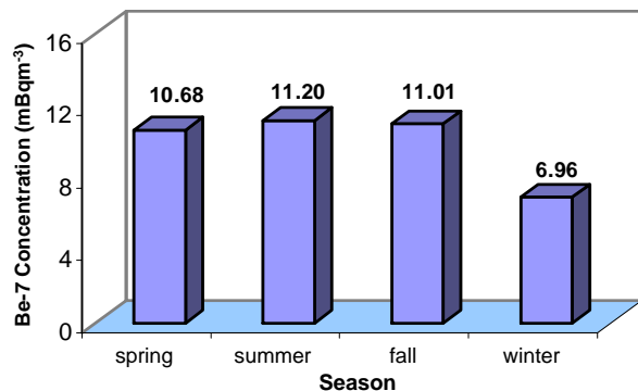
شکل ۲- تغییرات فصلی غلظت پرتوزایی {}^7\text{Be} ، سال ۱۳۸۰، ایستگاه تهران.
