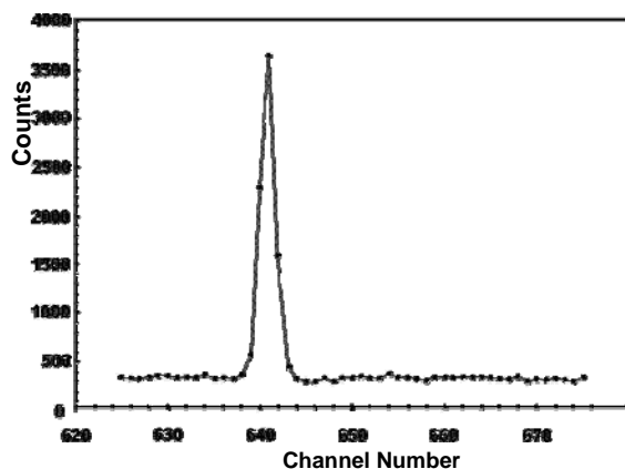
شکل ۱- طیف اسپکترومتری گامای رادیونوکلئید {}^7\text{Be} .
