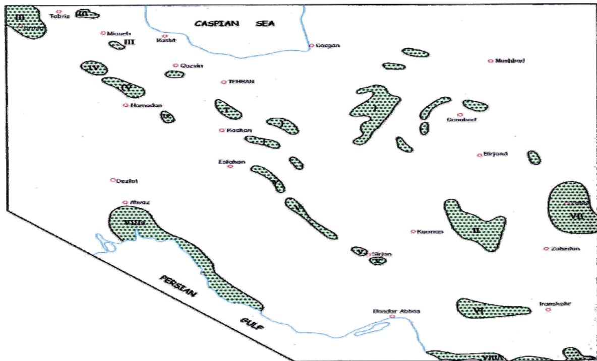
شکل ۱- نقشه ساده‌ای از حوضه‌های رسوبی جوان ایران.
