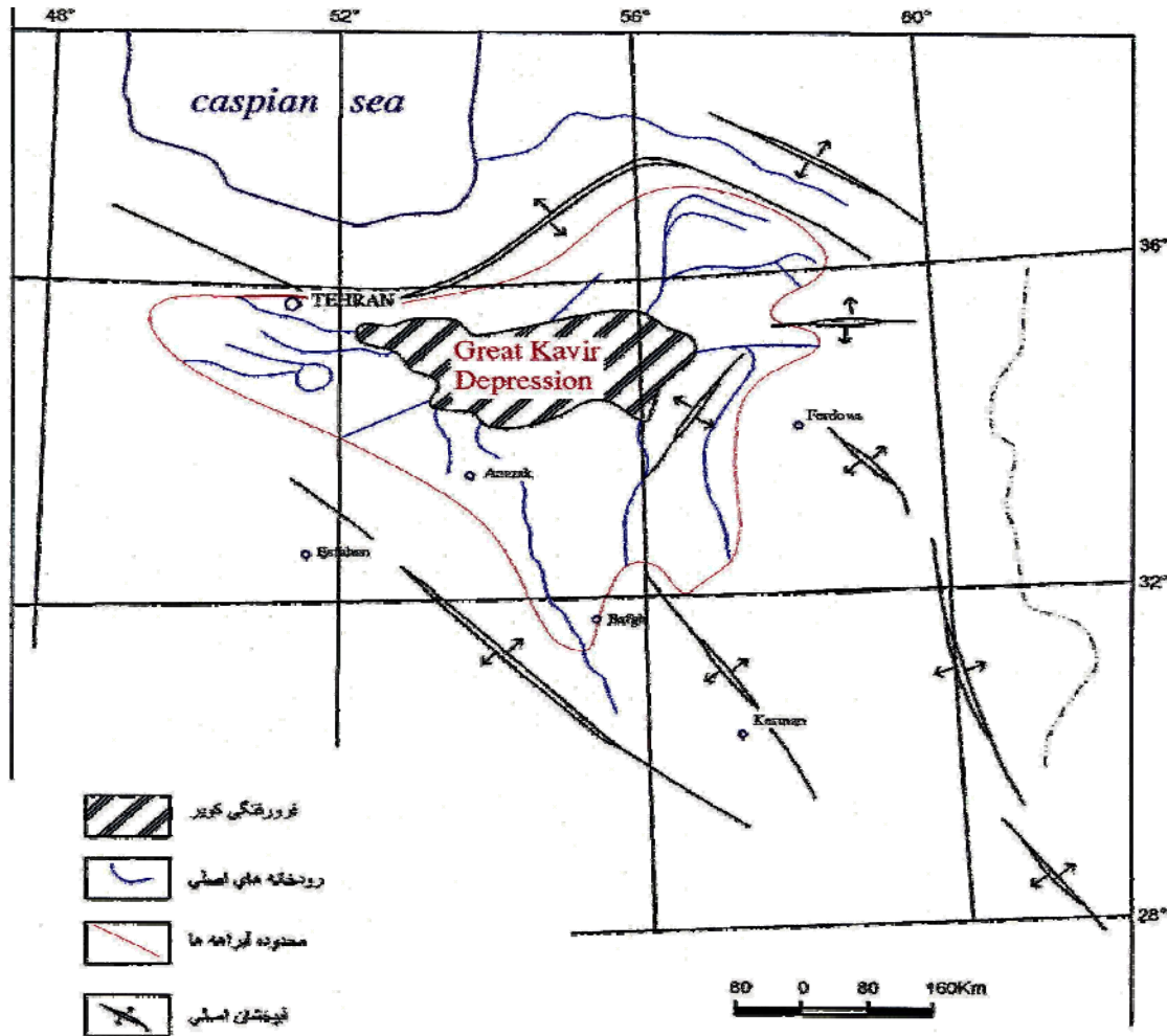
شکل ۲- نقشه ساده‌ای از فرورفتگی کویر بزرگ و سیستم آبراه‌های آن در الیگوسن - میوسن.
