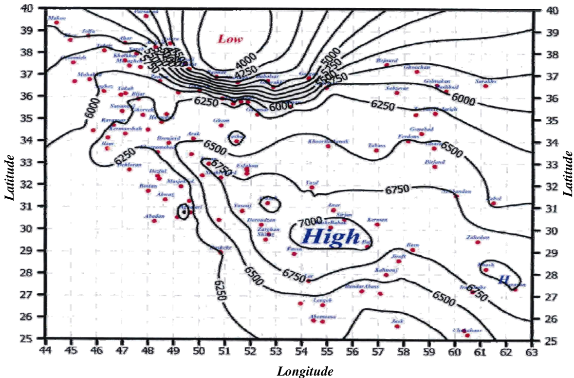
شکل ۱- مجموع انرژی تابشی کلی خورشیدی رسیده به واحد سطح افقی در طول سال برای نقاط مختلف ایران برحسب MJ/m 2 .
