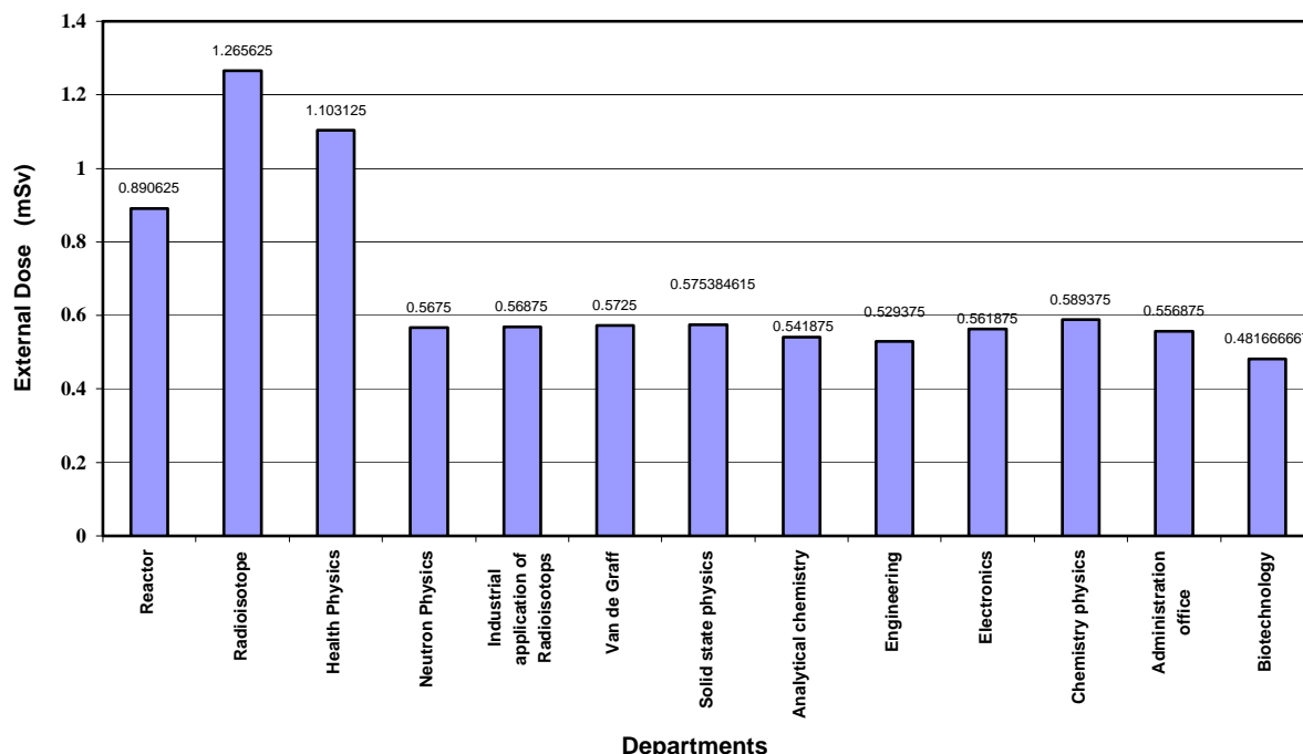
شکل ۲- نمودار میانگین مجموع دز خارجی دریافتی کارکنان بخشهای مختلف مرکز تحقیقات هسته‌ای طی سالهای ۱۳۸۲-۱۳۶۷.
