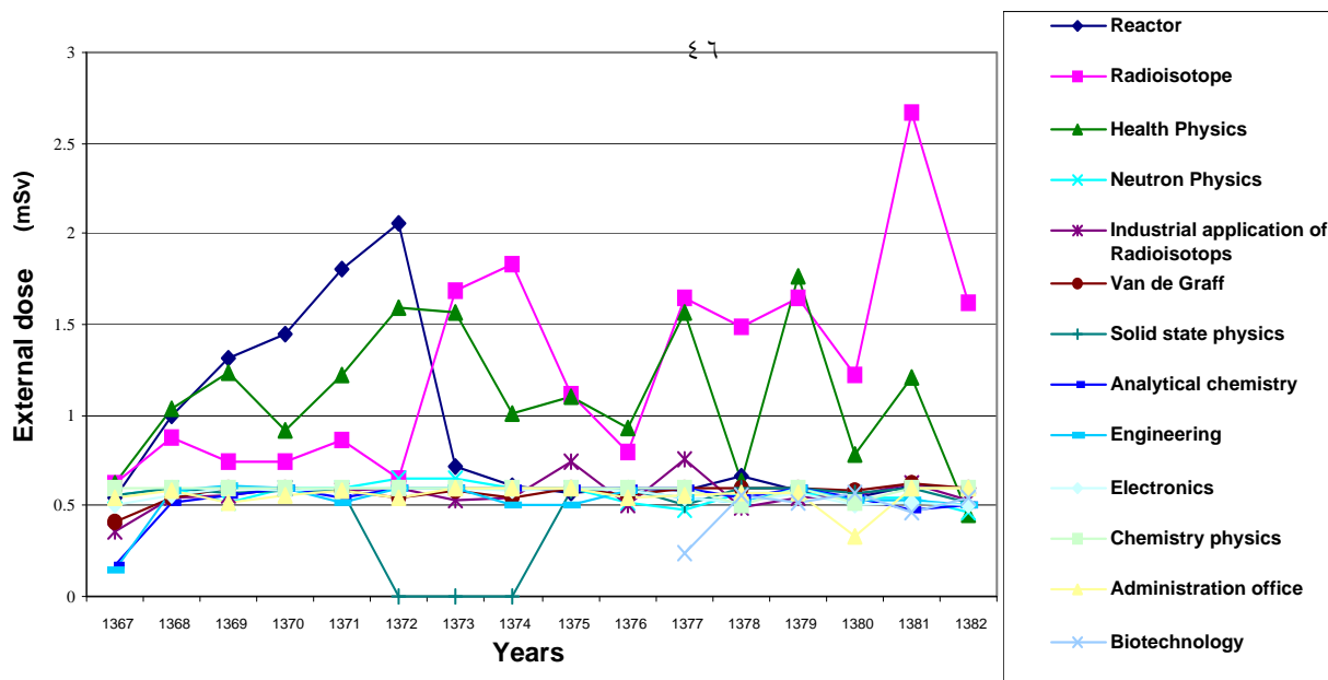
شکل ۲- نمودار میانگین مجموع دز خارجی دریافتی کارکنان بخشهای مختلف مرکز تحقیقات هسته‌ای طی سالهای ۱۳۸۲-۱۳۶۷.
