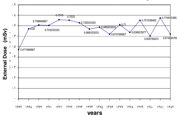
شکل ۱- نمودار میانگین مجموع دُز خارجی دریافتی کل کارکنان مرکز تحقیقات هسته‌ای طی سالهای ۱۳۶۷-۱۳۸۲.
