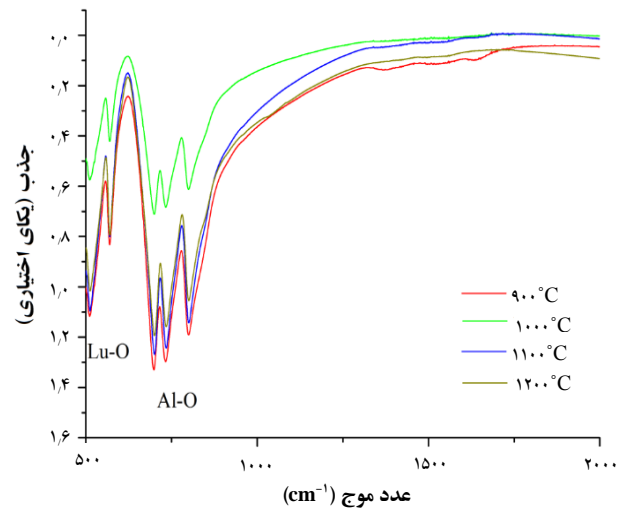
شکل ۳. طیف تبدیل فوریه ی زیرقرمز (FTIR) نانوبلورهای گارنت آلاییده شده با تربیم، تهیه شده در دماهای مختلف به روش هم رسوبی.
