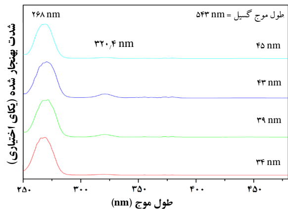
شکل ۶. طیف برانگیختگی بهنجار شده‌ی نانوبلورهای مختلف لوتسیم آلومینیم گارنت آلائیده شده با تربیم برای طول موج گسیل ۵۴۳ nm.
