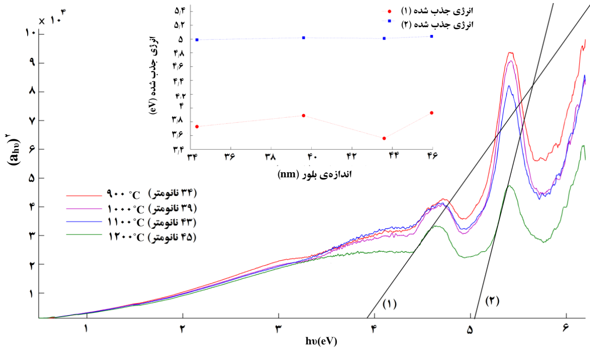
شکل ۴. طیف دیدگانی- فرابنفش و مقادیر انرژی جذب شده به دست آمده از نانوبلورهای مختلف لوتسیم آلومینیم گارنت آلائیده شده با تربیم.
