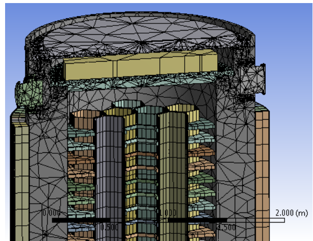
شکل ۵. مش‌بندی محفظه‌ی دومنظوره‌ی سوخت‌های مصرف‌شده‌ی رآکتور اتمی بوشهر به وسیله‌ی نرم‌افزار انسیس ورک‌بنچ.
