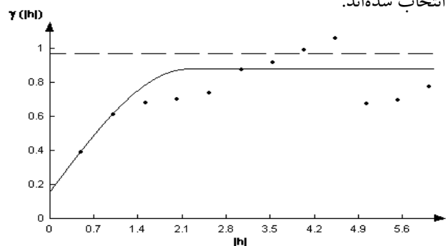
شکل ۶- تغییرنمای تئوری و تغییرنمای تجربی عیار اورانیوم در منطقه کم‌عیار
