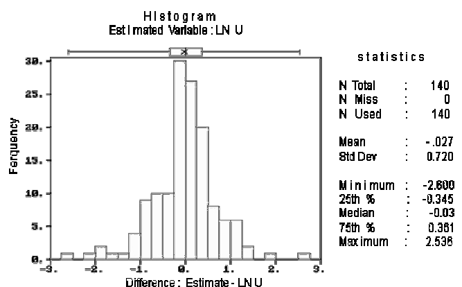
شکل ۷- نمودار ستونی خطاهای تخمین در منطقه کم‌عیار
