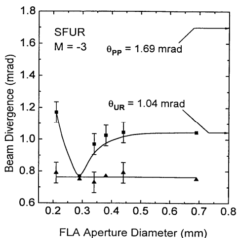
شکل ۸- تغییر واگرایی باریکه خروجی لیزر رزینه‌ای در راستای X و Y بر حسب تغییر اندازه روزه محدودکننده میدان.
