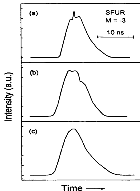
شکل ۷- رفتار زمانی پالس خروجی از لیزر رزینه‌ای در فواصل متفاوت عدسی استوانه‌ای (CL) از سطح رنگ: (a) در فاصله ۴/۹ cm، (b) در فاصله ۴/۸ cm، (c) در فاصله ۵/۲ cm.
