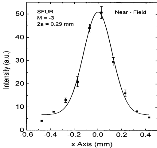
شکل ۴- نمودار توزیع گاوسی میدان نزدیک برای باریکه خروجی لیزر (در جهت x ).
