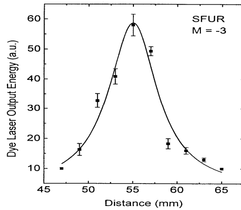
شکل ۲- تغییرات انرژی خروجی لیزر رزینه‌ای بر حسب فاصله عدسی استوانه‌ای تا سطح مایع رنگ.
