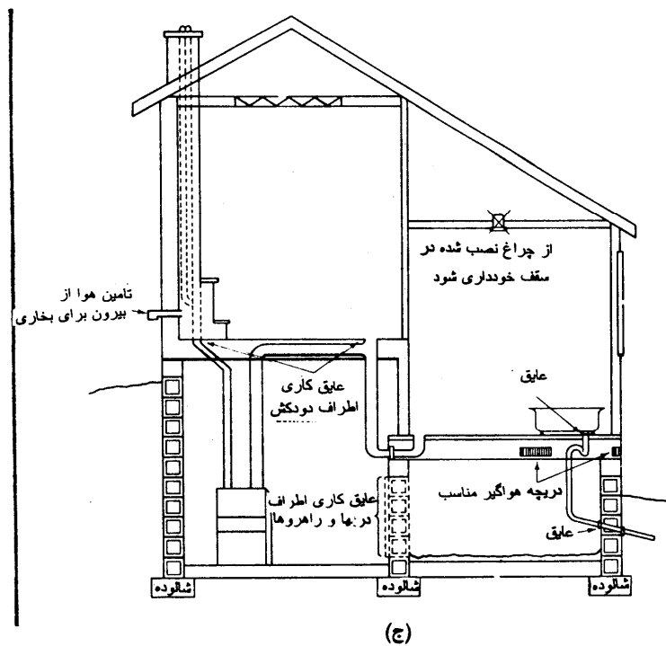
شکل ۵- روشهای کاهش مقدار رادون در ساختمان ها: الف) تقویت میزان تهویه زیرزمین ها، ب) ایجاد مکش در زیر کف ساختمان، ج) کاهش تاثیر تقلیل فشار هوا در ساختمان [۲۷].
